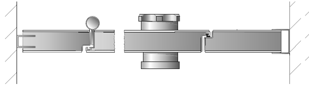
2 Schnitt Kabinenfront mit Einhandbeschlag Steigebändern aus Aluminium
