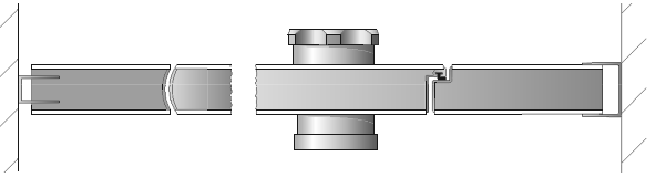
2 Schnitt Kabinenfront mit Einhandbeschlag und Aluminium-Fingerklemmschutz Scharnier optional
