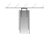
5 Wandanschluss optional als U-Profil mit Schattenfuge
