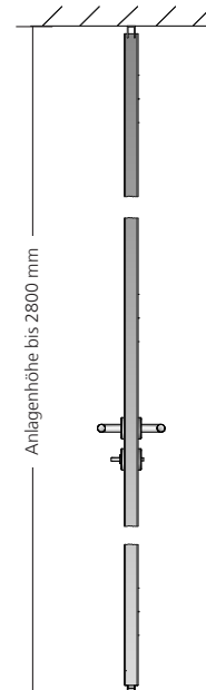
Höhschnitt Front
