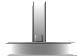
3 Anschluss Trennwand Front
